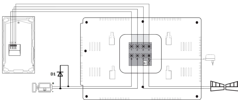
Diode D1= 1N4007
